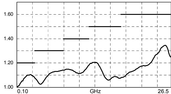
V.S.W.R.
