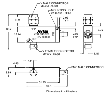
V251 outline
