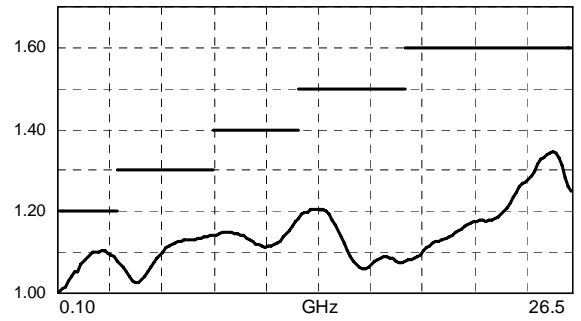
V.S.W.R.
